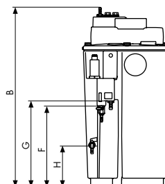
ÖWAMAT® 12-16 sans préséparateur
